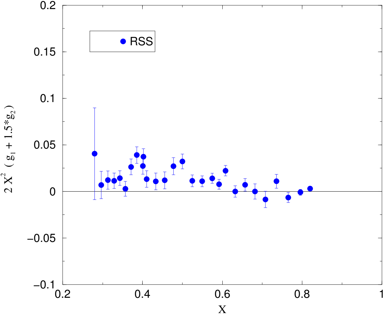
d 2 Integrand
