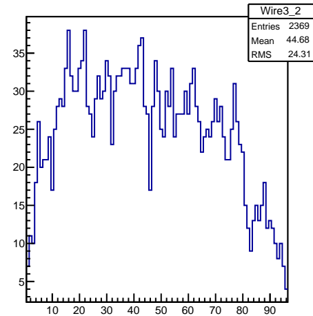
FDC4 Cell3 wire hits
