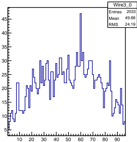
FDC4 Cell1 wire hits
