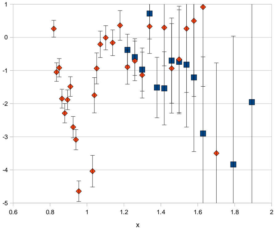
NH3 with right vnpol; ND3 with 43997 ◆ A para NH3 ■ A para ND3
