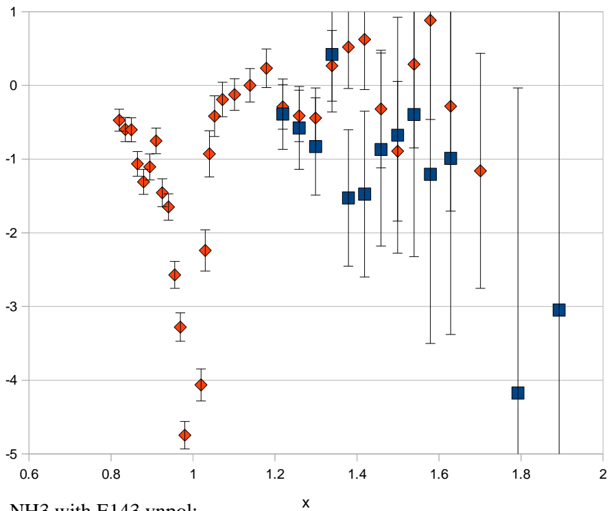
NH3 with E143 vnpol; ND3 no 43997 ■ A para ND3 ◆ A para NH3
