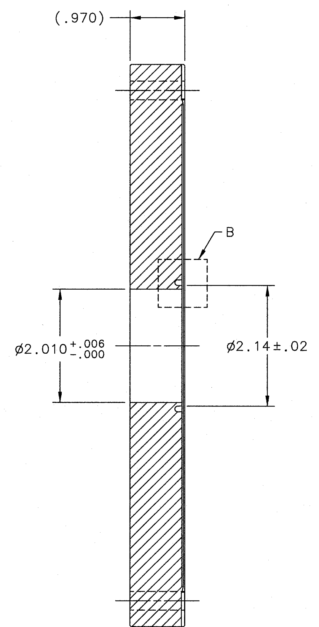
SECTION A-A
