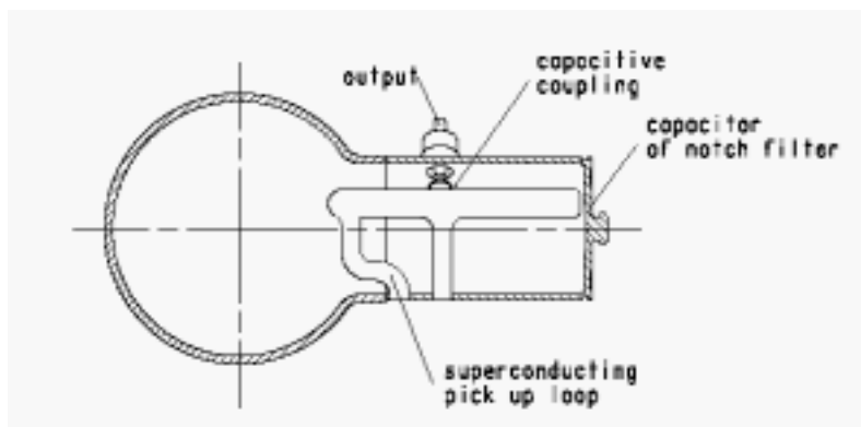
Fig. 5.2.3.1-6. The TESLA HOM coupler (TESLA 2001).
