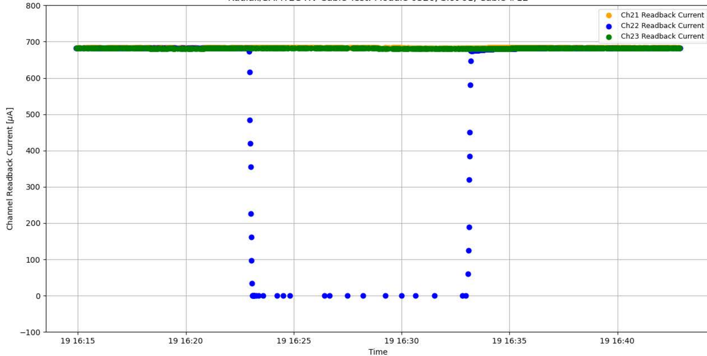
Radial/SAMTEC HV Cable Test: Module 0326, Slot 01, Cable #12
